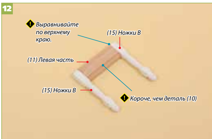
12 По обеим сторонам детали (11) прикрепите ножки В (15). ⚠ Выравнивайте по верхнему краю. ⚠ Короче, чем деталь (10)
