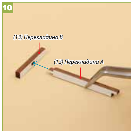
10 Вставьте выступ перекладины А в отверстие перекладины В, как показано выше. Прикрепите при помощи клея.
