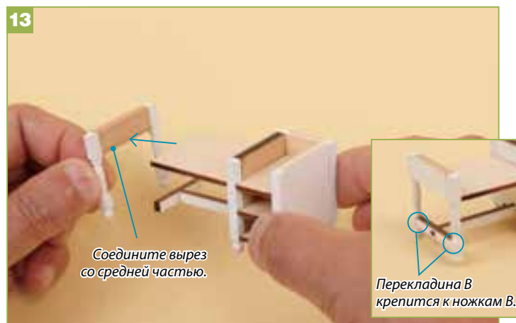
13 С левой стороны стола прикрепите левую боковину из шага 12. Соедините вырез со средней частью. Перекладина В крепится к ножкам В.
