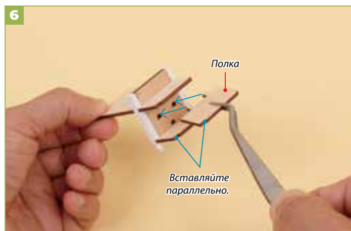
6 Аналогичным образом прикрепите при помощи клея вторую полку.
