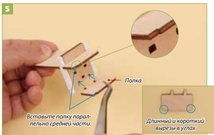
5 Вставьте выступы полки в отверстия в перегородке, закрепите при помощи клея для дерева.
