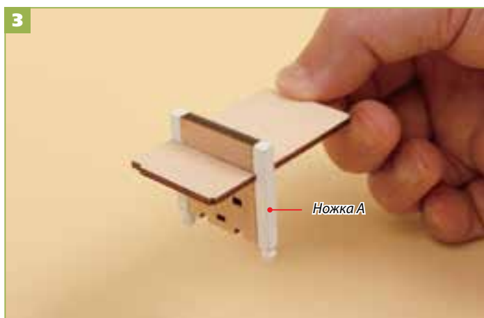
3 Аналогичным образом прикрепите с другой стороны перегородки вторую ножку А.
